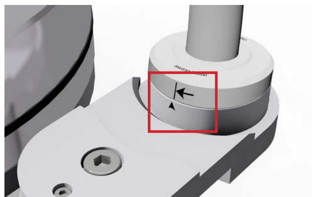
Abb. 14b: Montage der swing base (nach rechts)
